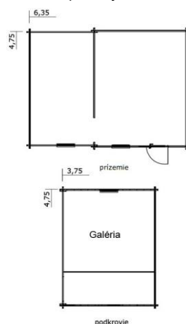
pôdorys
