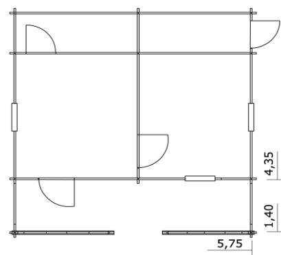
pôdorys
