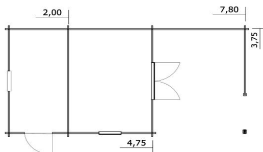
pôdorys
