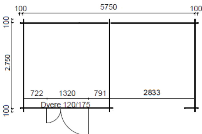
Pôdorys chatky:
