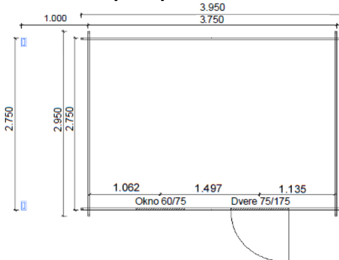
Pôdorys chatky:
