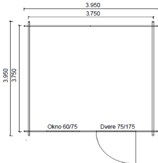
Pôdorys chatky:
