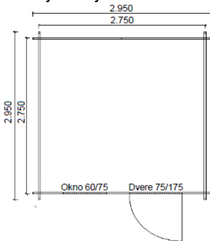
Pôdorys chatky:
