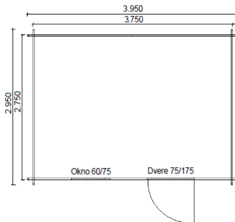
Pôdorys chatky:
