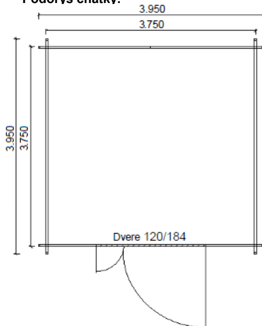
Pôdorys chatky:
