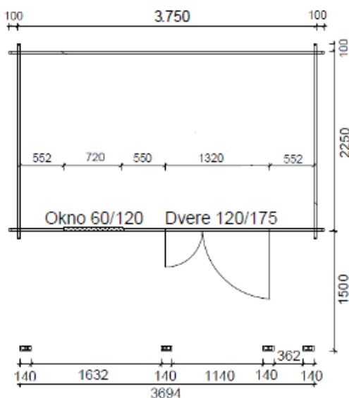
Pôdorys chatky:
