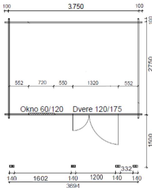
Pôdorys chatky:
