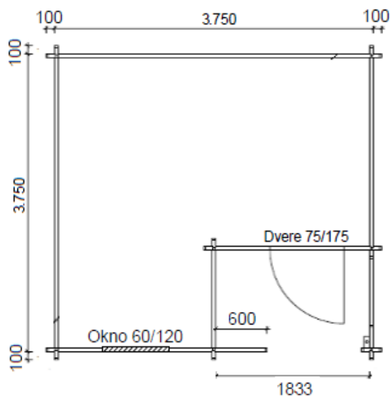
Pôdorys chatky:
